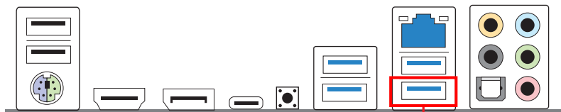
USB BIOS 回闪端口
