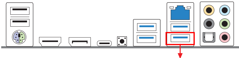
USB-BIOS-Flashback-Port
